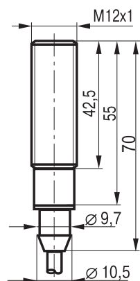
Габаритный чертеж
